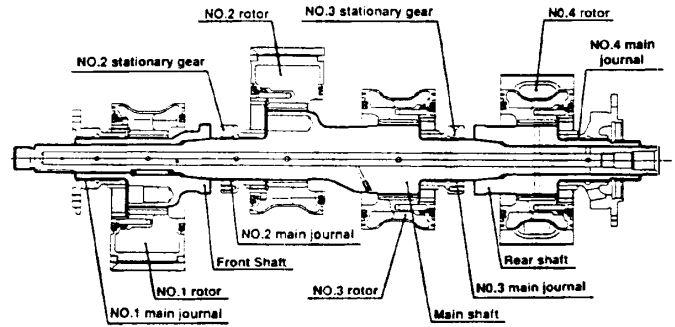
Fig. 7 Eccentric shaft
